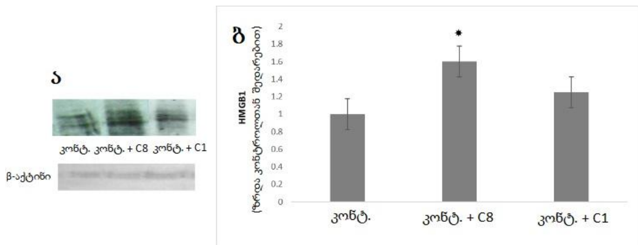
სურათი 22. RAW 264.7 მაკროფაგებში HMGB1-ის ექსპრესიის ცვლილება მფც-ს C8 და C1 იზომერების გავლენით. სამი დამოუკიდებლად ჩატარებული პარალელური ექსპერიმენტიდან მონაცემი წარმოდგენილია საშუალო \pm SEM-ით. * P < 0.05 საკონტროლო უჯრედებთან მიმართებაში.
