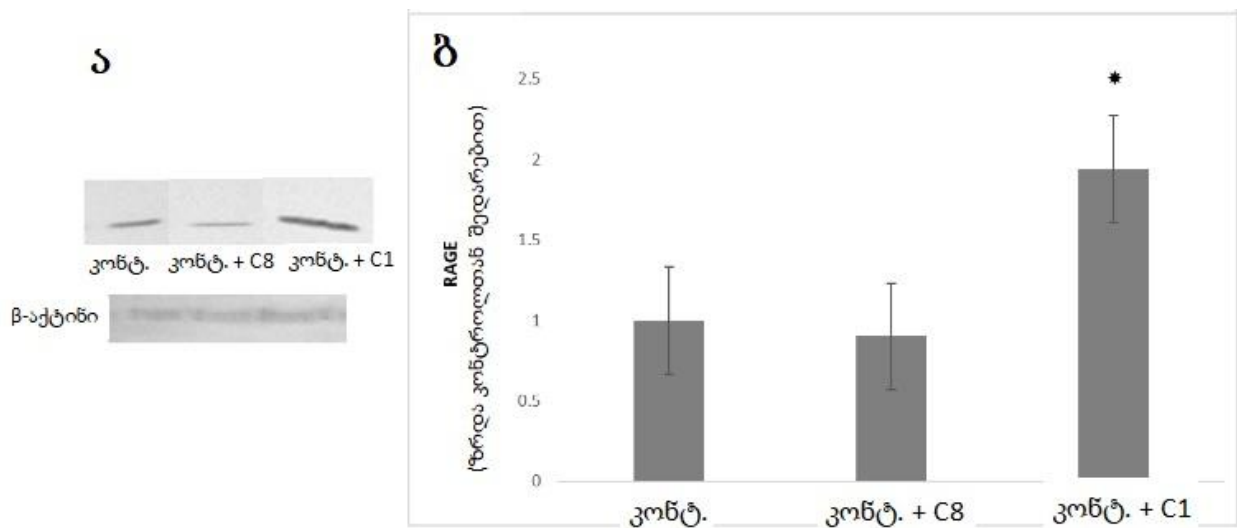
სურათი 23. RAW 264.7 მაკროფაგებში RAGE-ს ექსპრესიის ცვლილება მფც-ს C8 და C1 იზომერების გავლენით. სამი დამოუკიდებლად ჩატარებული პარალელური ექსპერიმენტიდან მონაცემი წარმოდგენილია საშუალო \pm SEM-ით. * P < 0.05 საკონტროლო უჯრედებთან მიმართებაში.
