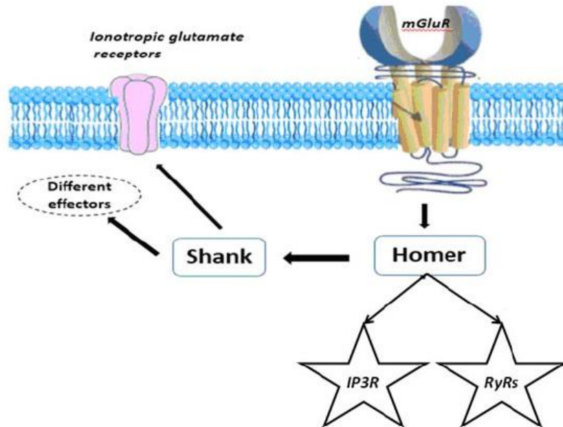
სურათი 5. mGluR-ის ურთიერთქმედება უჯრედშიდა სასიგნალო მოლეკულებთან.
