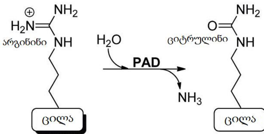
სურ. 2. არგინინის გარდაქმნა ციტრულინად ფერმენტული სისტემის პეპტიდილ-არგინინ დეიმინაზას მოქმედებით.
