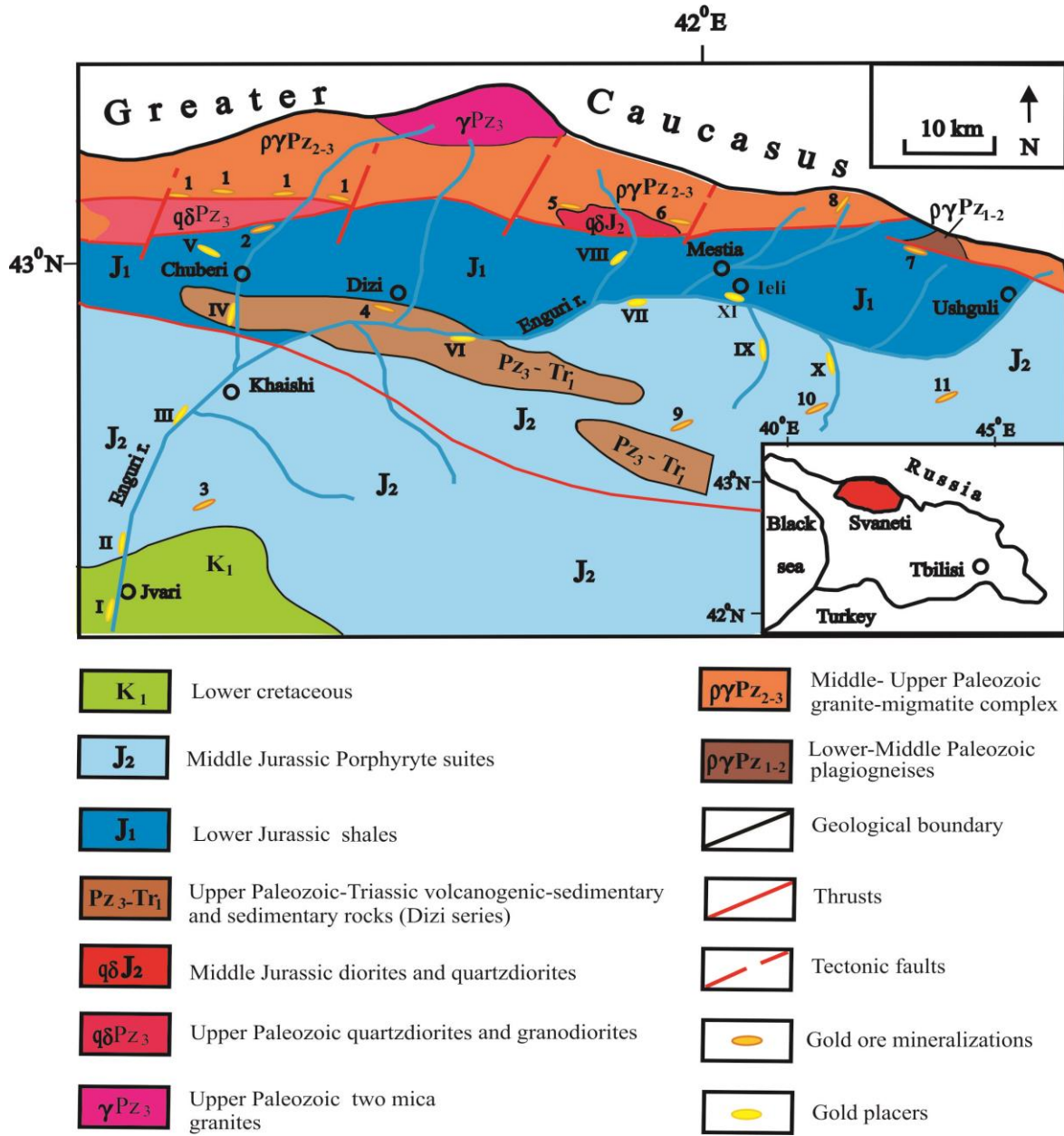
ნახ. 4. სვანეთის სქემატური გეოლოგიური რუკა, რომელზედაც დატანილია ოქროს ძირითადი და ქვიშრობული გამადნებები.
